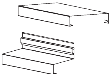
Detail RHEINZINK-Abdeckungen für den Dachrand
