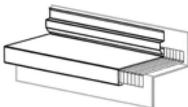
Detail Stoßbereich Gesimsabdeckung mit Kapleiste und UDS-Verbinder
