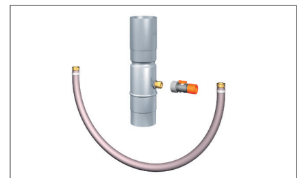
Regensammler mit GARDENA® Regulierstop (1/2 Zoll) und Verbindungsschlauch (1 Zoll) für den Direktanschluss an eine Regentonne
